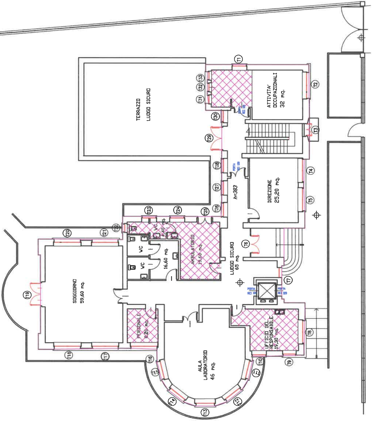
PIANTA PIANO TERRENO
